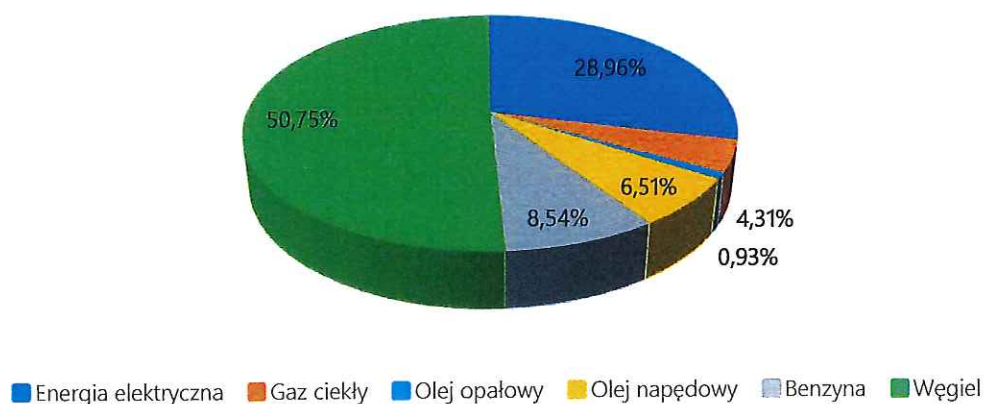
Wykres 10. Udział paliw w bilansie emisji dwutlenku węgla na terenie gminy Białobrzegi. Źródło: Opracowanie własne.
